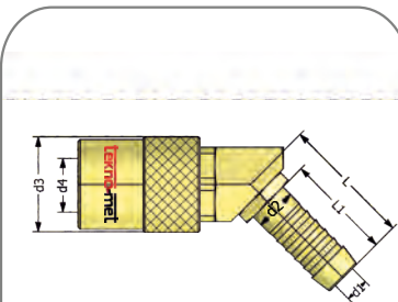
Standard hose tail socket 45° Kupplung mit 45° Standard-Schlauchtülle
