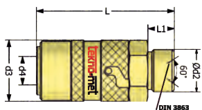
Parallel Male Thread Kupplung mit Aussengewinde
