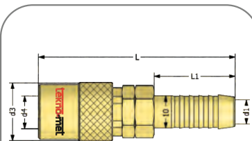
Standard hose tail socket Kupplung mit gerader Standard-Schlauchtülle
