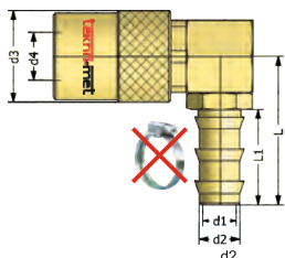
Standard hose tail socket 90° Kupplung mit 90° Schnellsteck-Schlauchtülle
