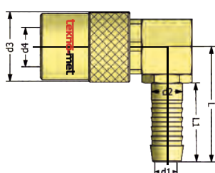
Standard hose tail socket 90° Kupplung mit 90° Standard-Schlauchtülle
