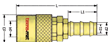
Push-Lock hose tail socket Kupplung mit gerade Schnellsteck-Schlauchtülle
