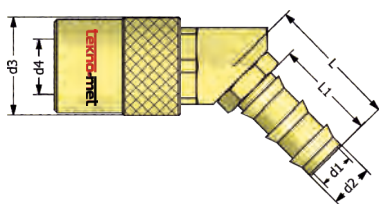
Push-Lock hose tail socket 45° Kupplung mit 45° Schnellsteck-Schlauchtülle
