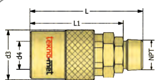
NPT Thread socket Kupplung mit Aussengewinde NPT
